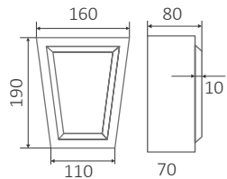
Оконный наличник угловой левый 004/2
