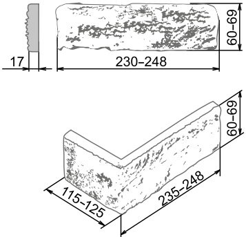
Тычковые элементы «Марсель»
