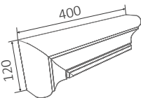
Оконный наличник прямой 004
