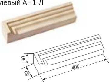
Наличник угловой левый АН1-Л
