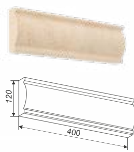
Наличник прямой АН3
