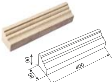
Наличник прямой АН1
