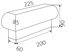
Подоконник угловой левый 006/2
