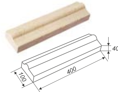
Карниз прямой АК2
