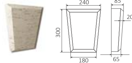
Дверной наличник угловой левый 005/2
