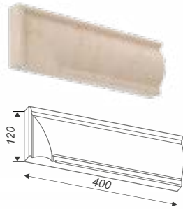
Наличник угловой левый АН3-Л
