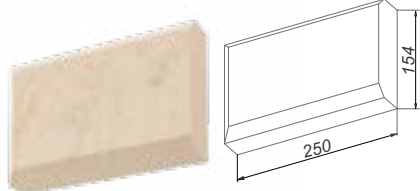
Рустовой камень обрезной АР1-ОБР
