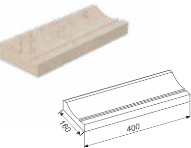
Наличник прямой АН3
