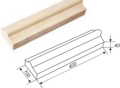
Карниз угловой правый АК1-П
