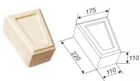
Замковый камень АЗ-1
